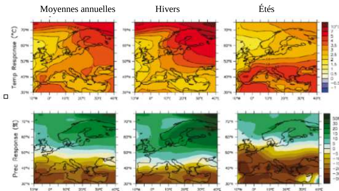
Figure 8. Changements de températures et de précipitations 1980-2000/2080-2099 (scénario A1B du GIEC)
