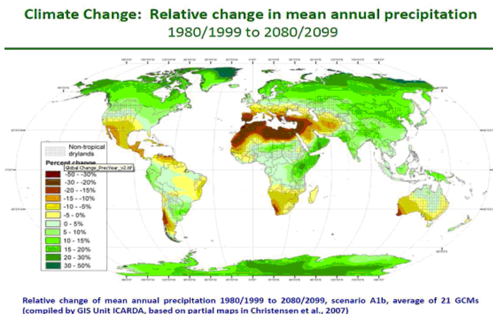
Figure 7 : changements annoncés de la pluviométrie sur un siècle : la Méditerranée site critique mondial
