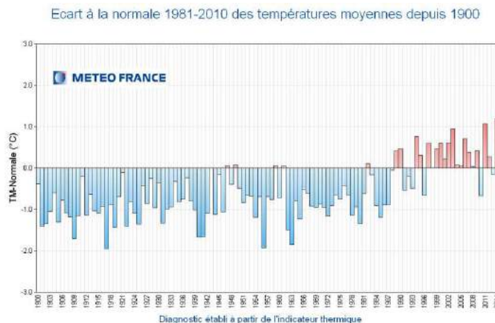
Figure 10 : Le réchauffement climatique en France
