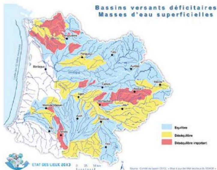
Figure 23 : Bassins versants déficitaires et écarts entre volumes « prélevables » et volumes prélevés : Sud-Ouest
