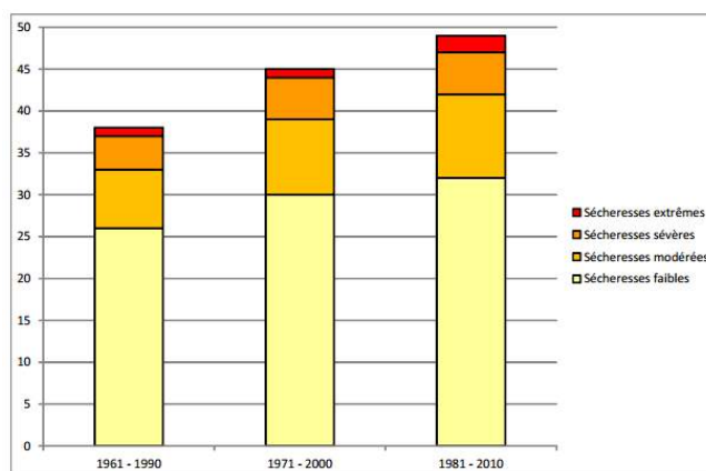
Figure 15 : Sévérités des sécheresses à 3 mois dans la Vienne 1960-2010 (% du temps) 20
