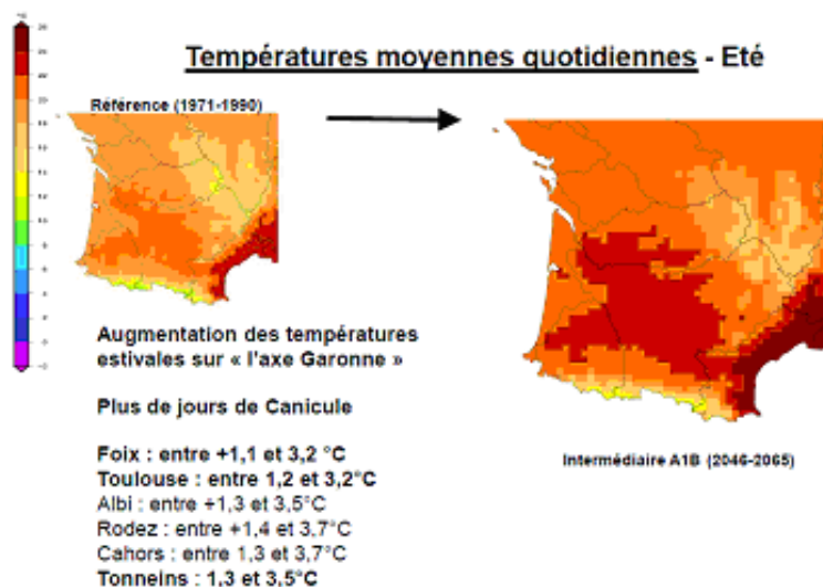
Figure 41 : Évolution des températures moyennes quotidiennes en été d'ici 2050 dans le Sud Ouest
